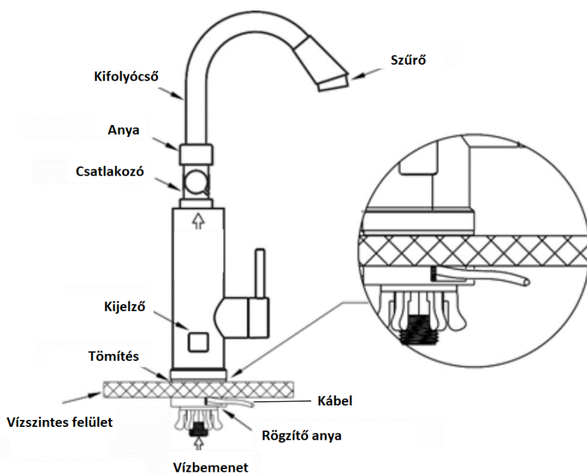
2. ábra. Tápkábel kimenete a mosogató alatt
