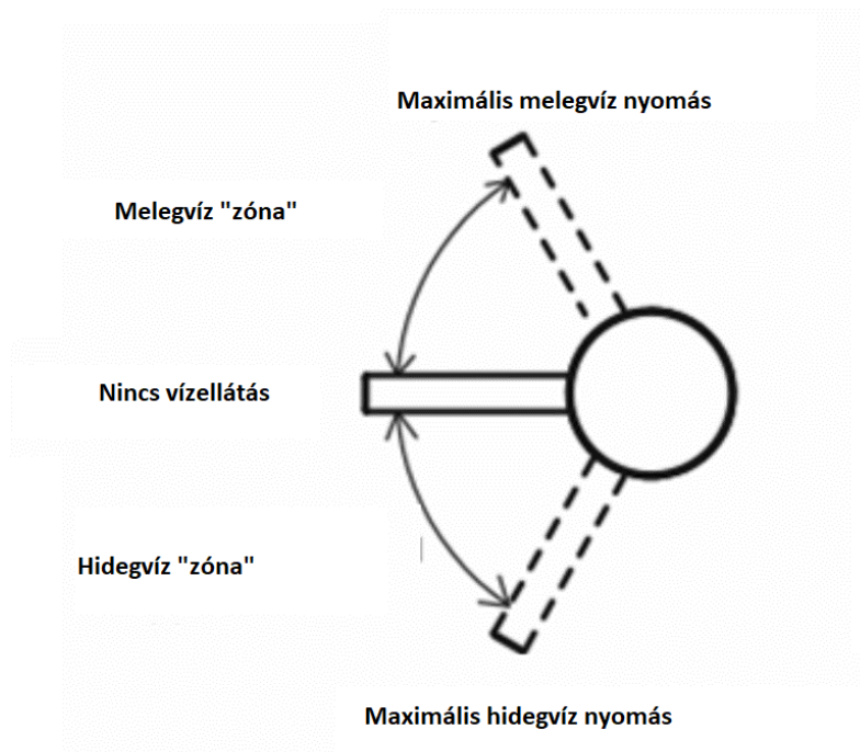
3. ábra A maximális vízhozam szabályozása.
